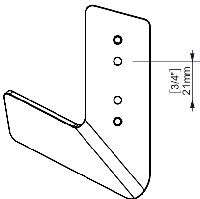
INSTALACIÓN PARED WALL FIXATION
