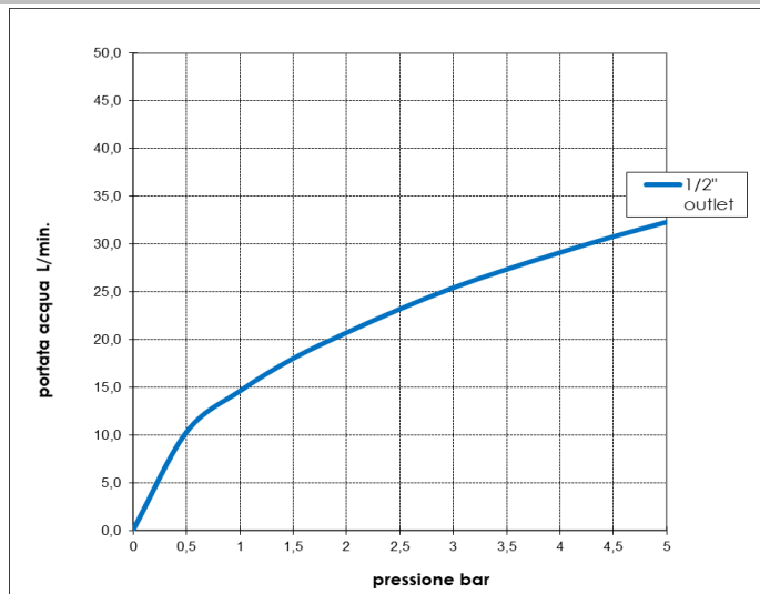
Grafico di portata - Flow rate diagram
